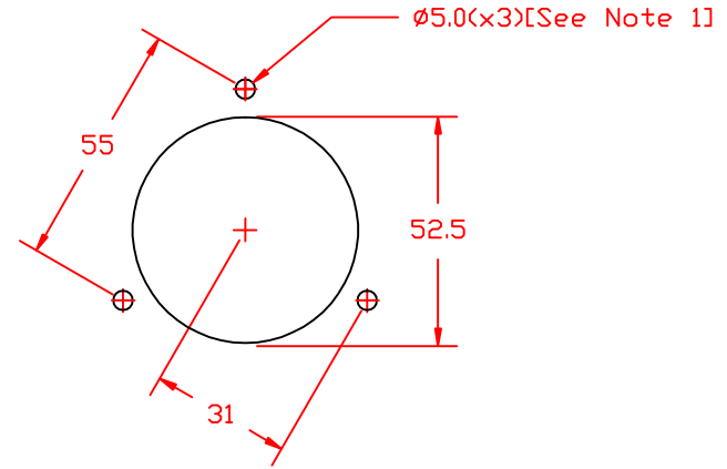
CUTOUT
